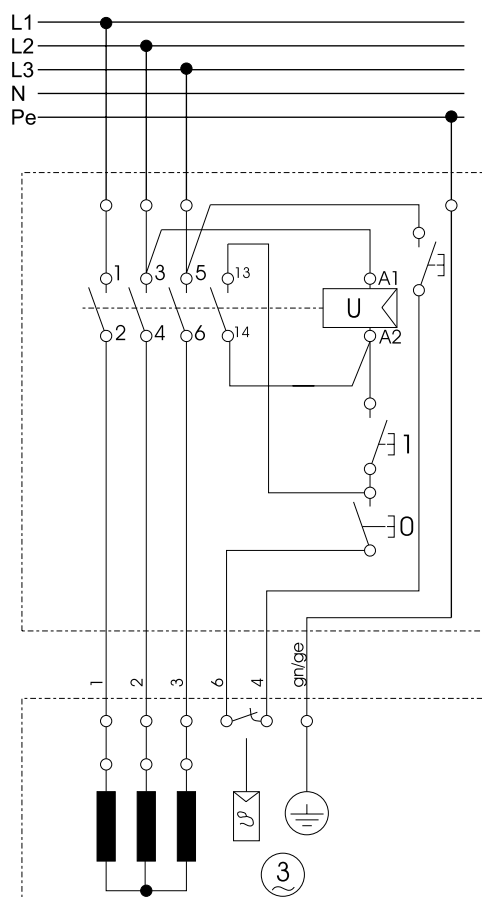
(7) Schéma du circuit
