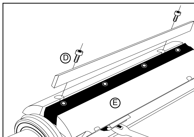
Montage du fer à raboter dans le porte-outils.
