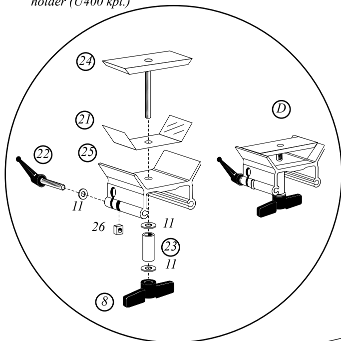
Front guide rail holder (U400 kpl.)
