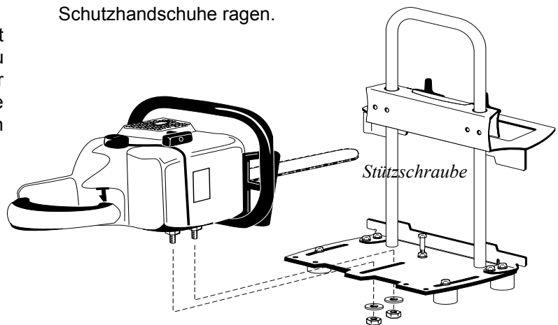
Original Kettensägen Schienenmutter mit Unterlagsscheiben (11x28x2).
