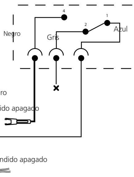
Interruptor de seguridad
