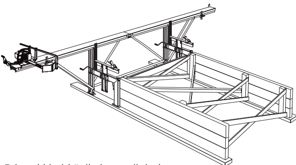
Esimerkki pitkäaikaiseen sijoitukseen tarkoitetusta tukkitasosta. LOGOSOL F2:een on saatavana lisävarusteena teräksiset tukkiportaat.
