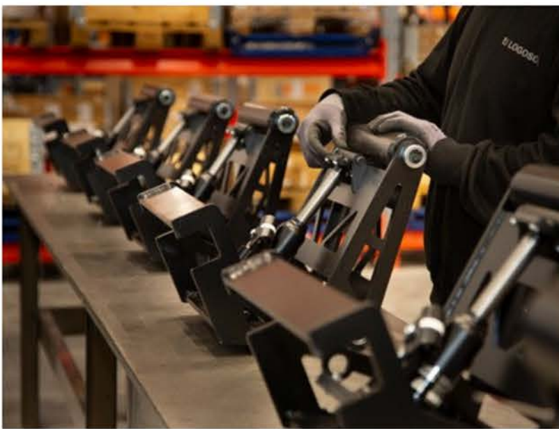
• Assemblage à la chaîne des correcteurs de conicité pour scierie à bande
