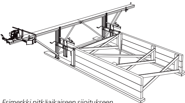
Esimerkki pitkäaikaiseen sijoitukseen tarkoitettusta tukkitasosta. LOGOSOL F2:een on saatavana lisävarusteena teräksiset tukkiporta.
