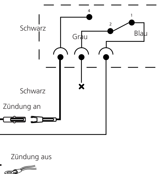
Interlock Sicherheitsschalter für den Schutzdeckel
