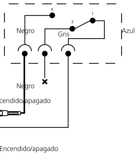
Interruptor de seguridad
