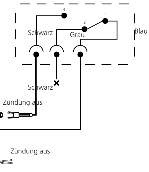
Sicherheitsschalter
