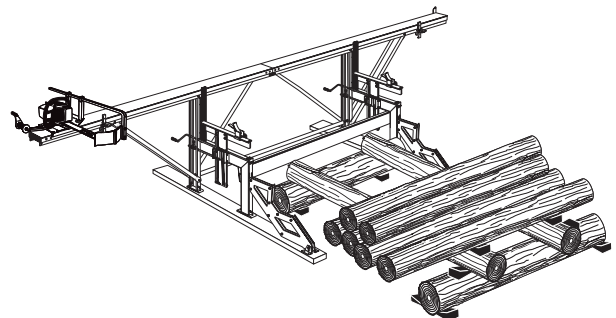
Exemple de table à grumes temporaire.
