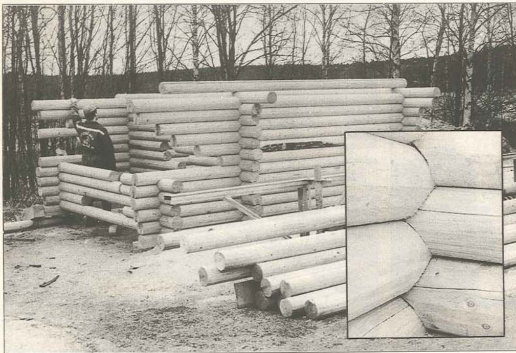
Den här stugan byggs med Solosågade stockar. Såväl "svartningen", knutarna och draget, ett spår under stockarna för tätning, har gjorts i sågverken med tillsats som är under utveckling. Den infällda bilden visar knuten i närbild.
