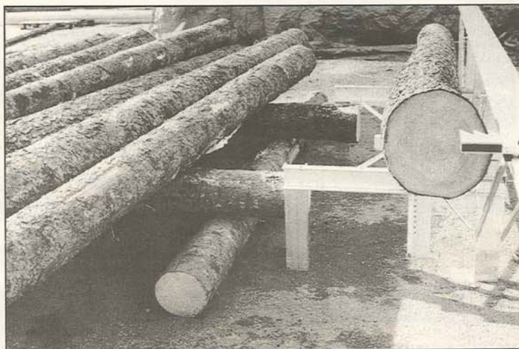
Ett stockbord gör sågningen effektiv. Man kan bygga det av plank eller, som på bilden, lägga ihop några stockar. På bilden i nedanstående artikel ser du skytten av ett stockbord av plankor.
