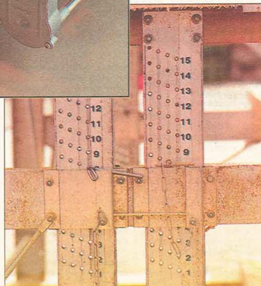
En vanlig Solosåg klarar galant stockar på 500 kg enligt Statens Maskinprovningar. För den som arbetar med riktigt grovt timmer finns en förstärkningstillsats med dubbla hålskivor och längre stockhyllor. Du kan köpa din Solosåg direkt i förstärkt utförande eller bygga om den i efterhand.
