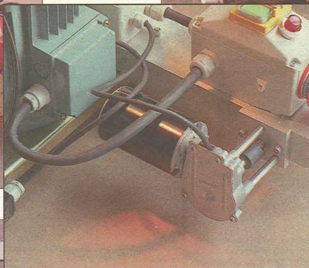
Solosågen kan förlängas i fyra steg. 0,5, 1 och 2,5 meter extra. Eller med en sågbänk till.
