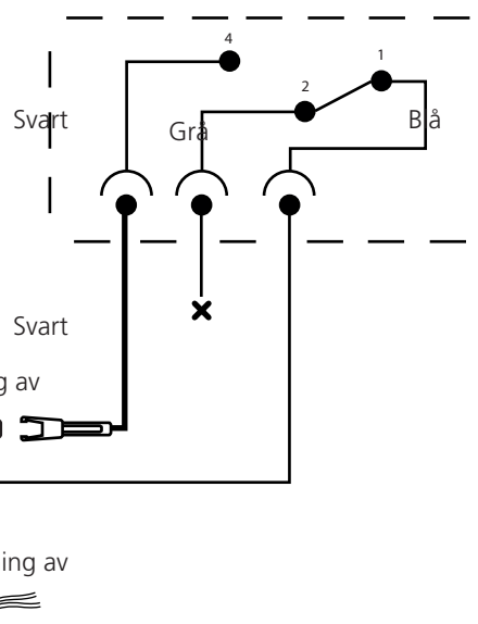
Sikkerhetsbryter
