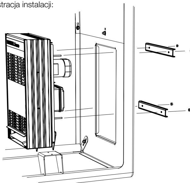
Ilustracja instalacji:
