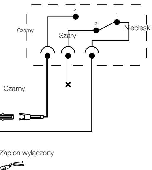
Wyłącznik bezpieczeństwa
