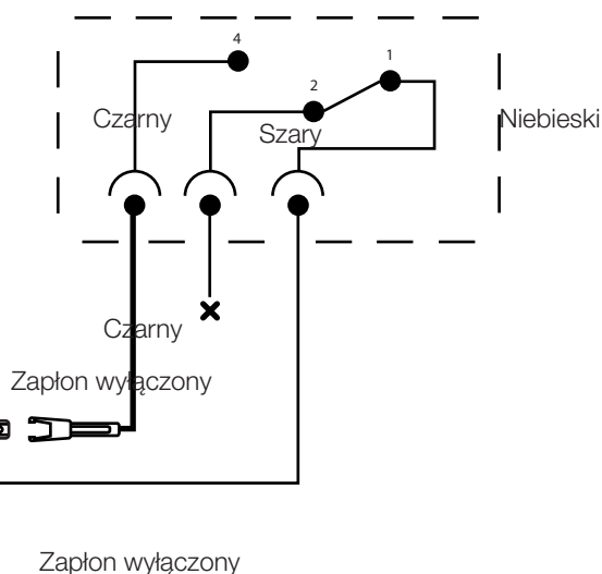
Wyłącznik bezpieczeństwa
