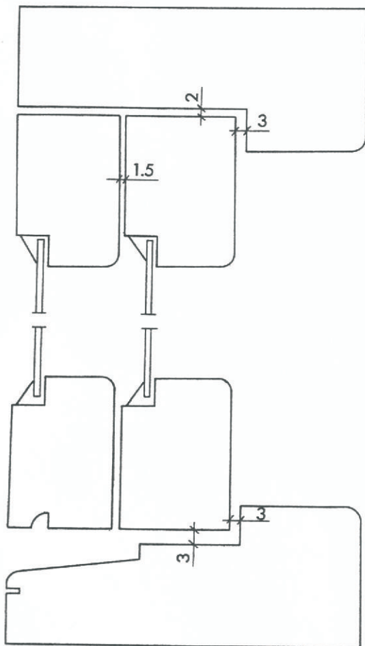
Vertikalsnitt
