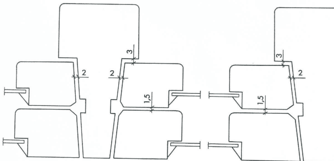
Horizontalsnitt
