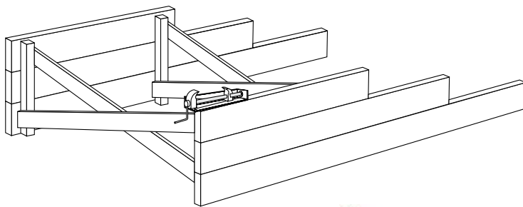
Stockhållare
