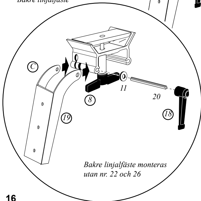
Bakre linjalfäste
