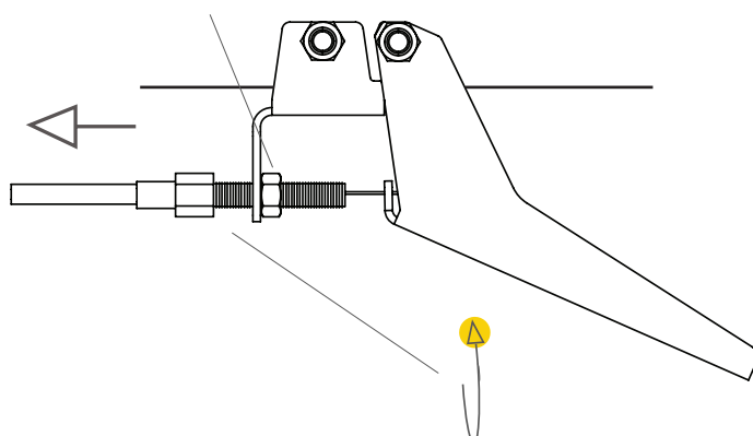
Kontramutter
