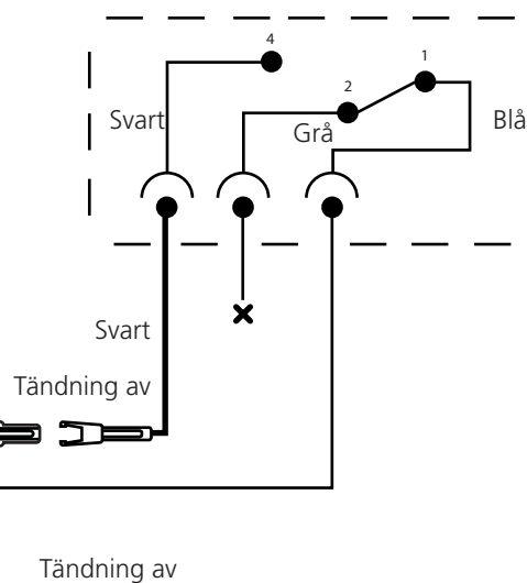
Säkerhetsbrytare
